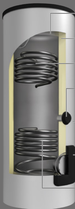
Logalux ESM300 ES-B
