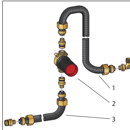
Abb. 1: Bauteile
