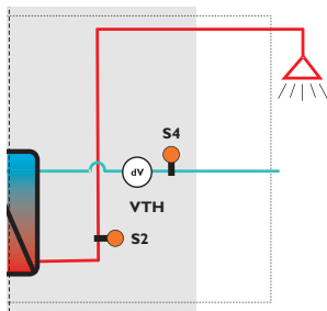
Sekundärseite
