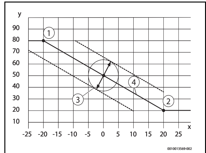
Bild 5 Außentemperaturgeführte Heizkurve
