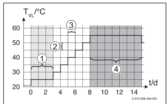
Bild 10 Ablauf der Estrichrocknung mit den Grundeinstellungen in der Aufheizphase
