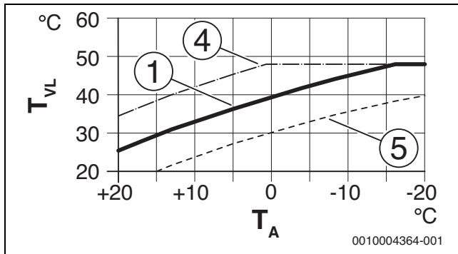
Bild 9 Einstellung der Heizkurve für Fußbodenheizung Parallelverschiebung über Raumtemperatur-Offset oder gewünschte Raumtemperatur
