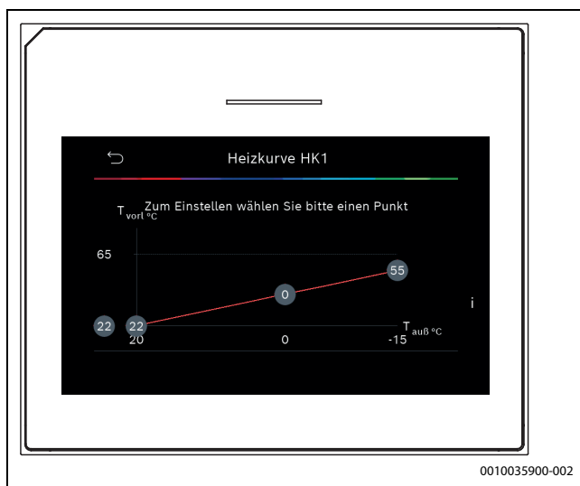
Bild 6 Endpunkt einstellen (Heizkurve Außentemperaturgeführt)
