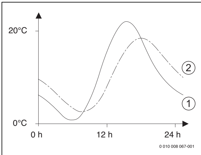
Bild 4 Beispiel für die gedämpfte Außentemperatur
