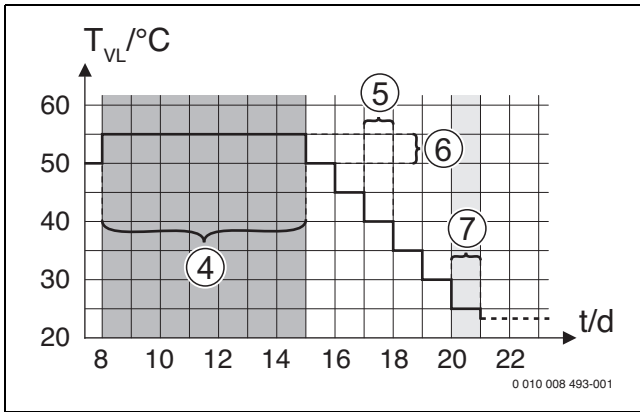
Bild 11 Ablauf der Estrichrocknung mit den Grundeinstellungen in der Abkühlphase
