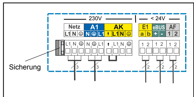
Bild: Sicherungswechsel
