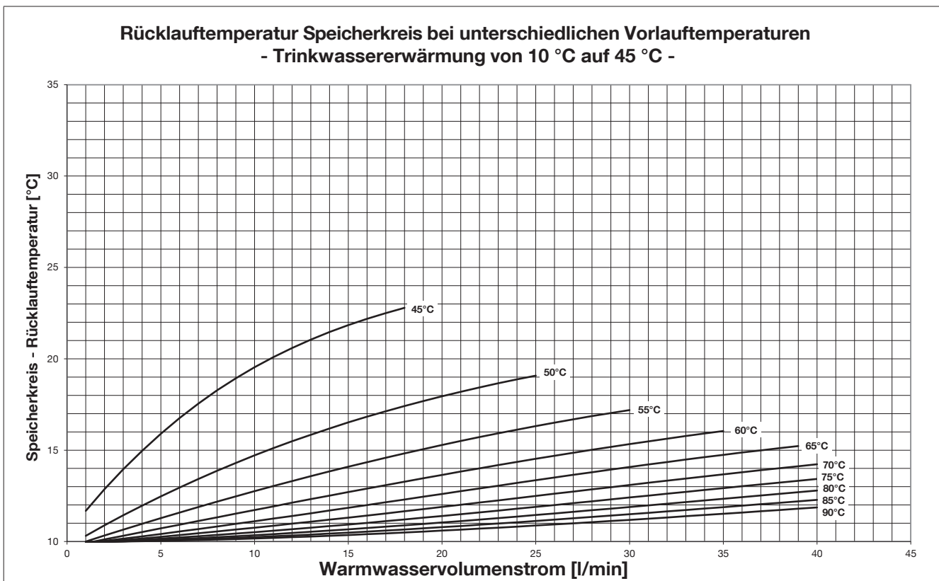
Abb. 7: Rücklauftemperatur Speicherkreis - Trinkwassererwärmung auf 45 °C
