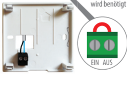
An WW-Timer angeschlossener Zylinderthermostat
