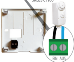
An Klemmleiste angeschlossener Zylinderthermostat (Standard)
