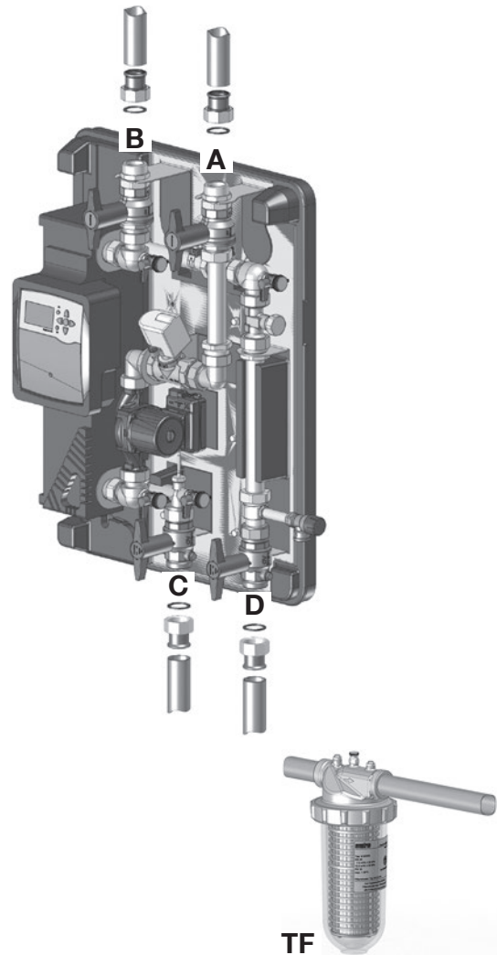
Abb. 4.8: Rohrleitungen mit Trinkwasser-Filter an Station anschließen
