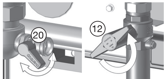
Abb. 5.10: Speicherkreisseite entlüften
