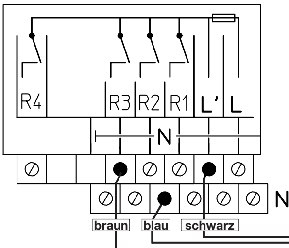
Abb. 4.11: Verdrahtung Stellmotor der Absperrereinheit mit dem Regler
