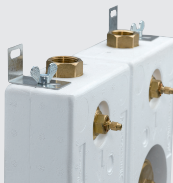
Befestigungsdarstellung Montagewinkel
