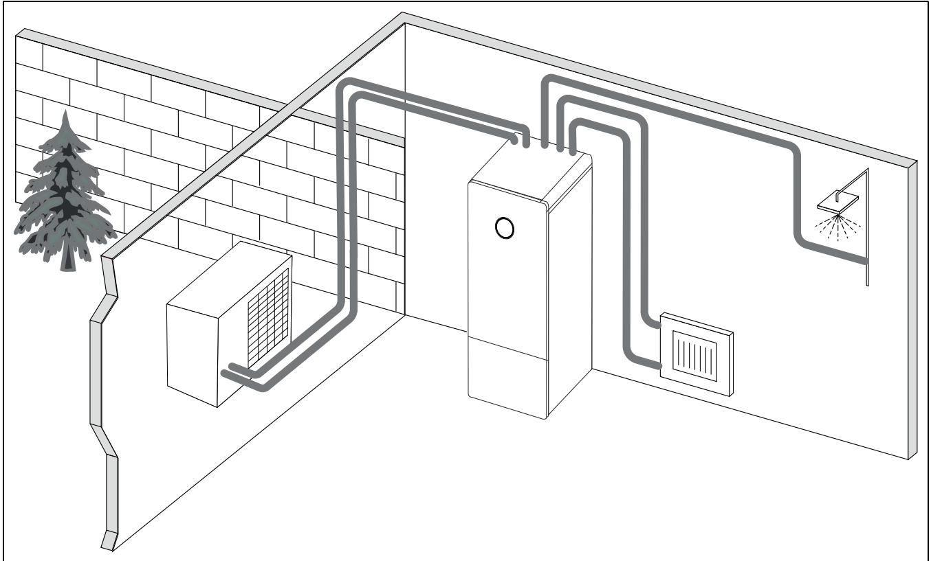
Bild 7 Wärmepumpe AW OR, Inneneinheit Compress 5800/6800i 12 M mit integrierter Warmwasserspeicher und elektrischem Zuheizung
