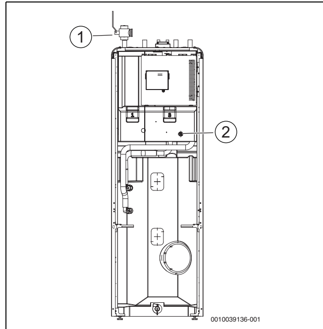
Bild 13 Compress 5800/6800i 12 M
