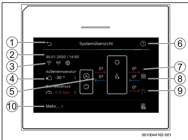
Bild 12 Systemübersicht
